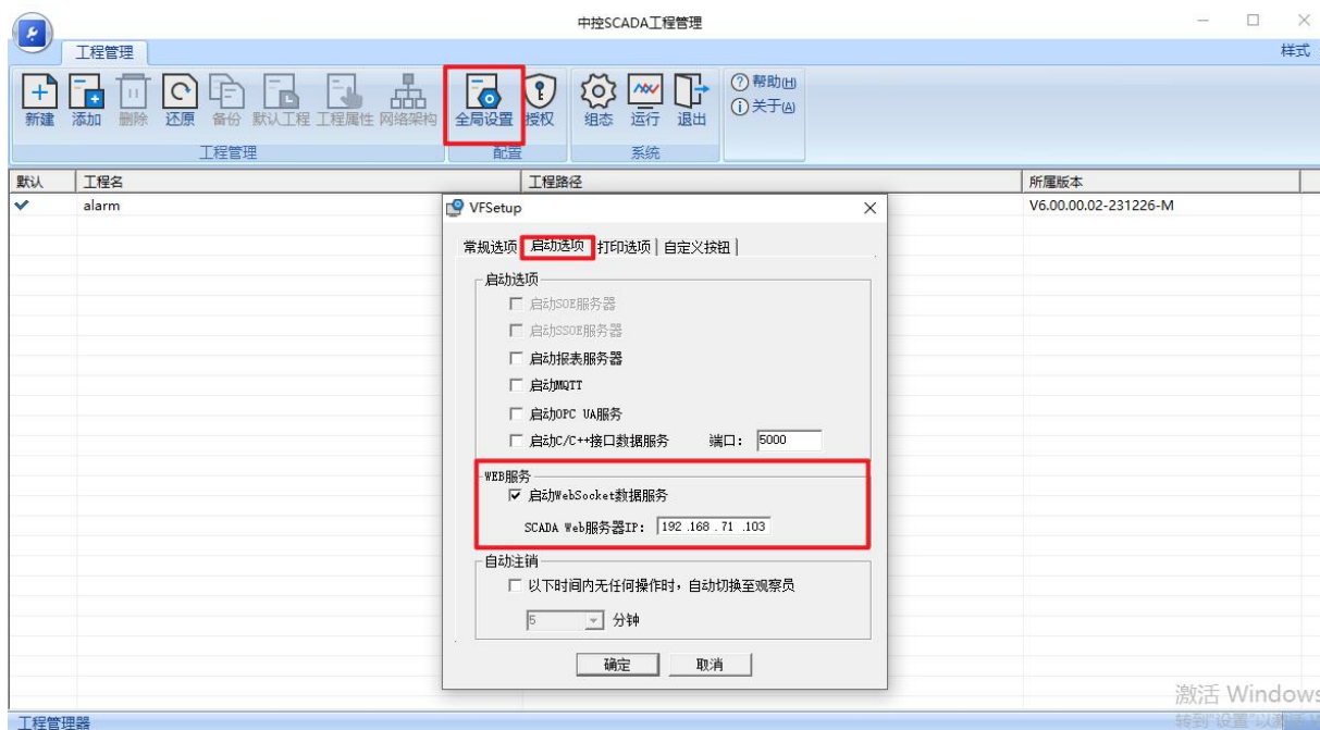
图 7-1 启动 WebSocket 服务
